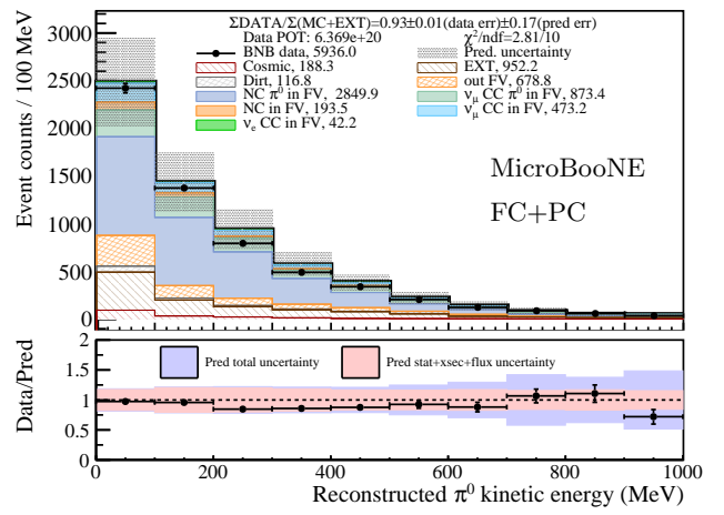
(d) NC\pi^0 reconstructed \pi^0 kinetic energy
