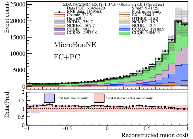
(d) Muon \cos\theta , broken down with interaction types
